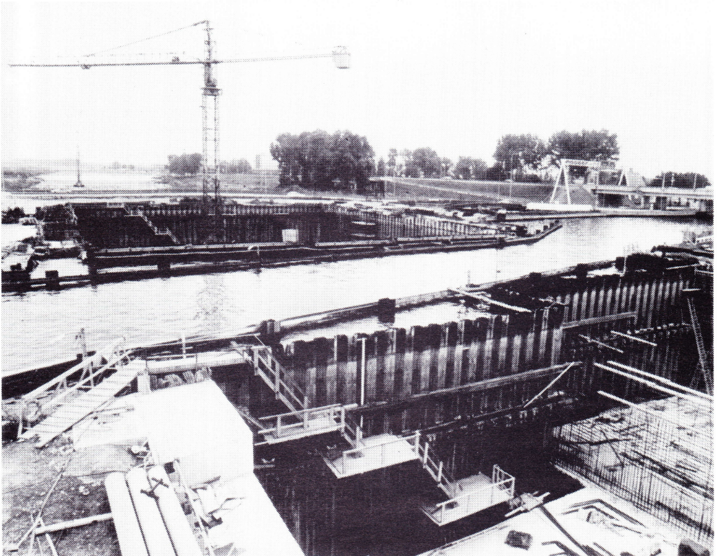
Er werd gewerkt met twee bouwputten. (Fotocollectie: SAMH)
