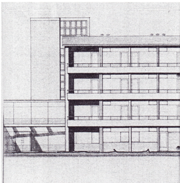
Tekening van een gedeelte van de oostgevel volgens de bestektekening uit juli 1959. (Archief Hervormde Gemeente Waddinxveen)
